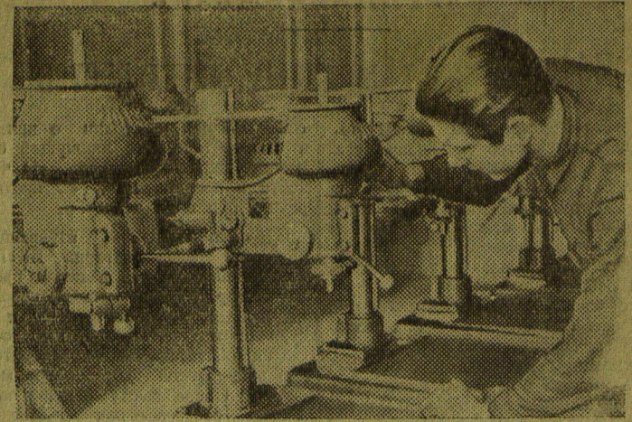
ЛИТОВСКАЯ ССР. Первенец послевоенной Сталинской пятилетки в Литве станкостроительный завод «Жальгирис» выпустил первые настольно-сверлильные станки. На снимке: слесарь Б. Гележаускас за регулировкой станка. Фото Л. Мейнерта. Прессклише ТАСС.
